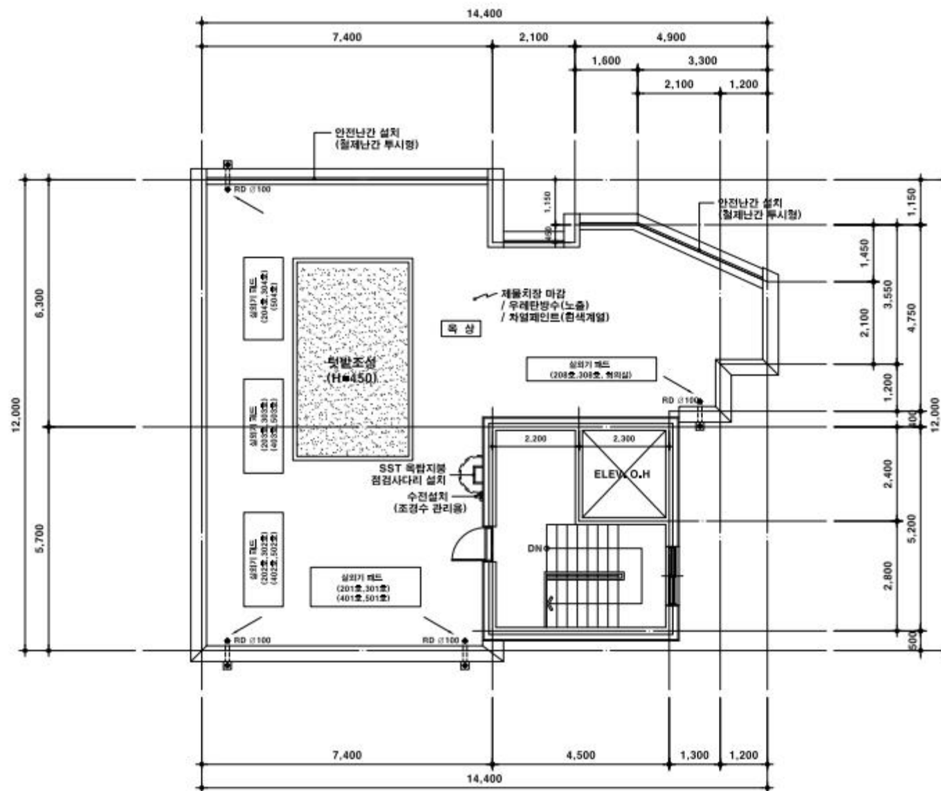
지붕 평면도 SCALE : 1 / 100
